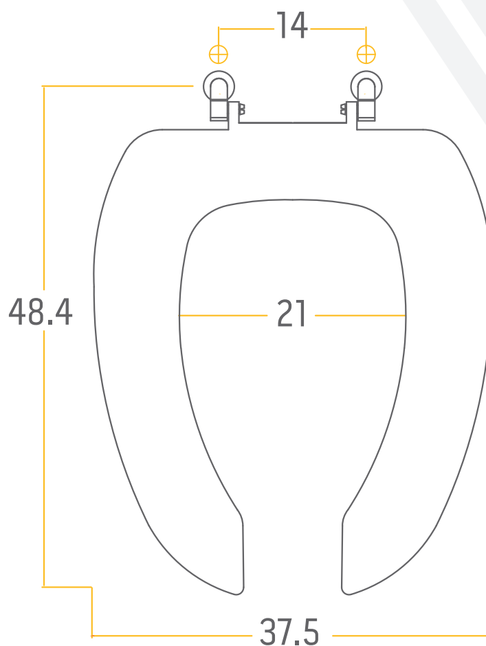
DIMENSIONES / VISTA SUPERIOR
