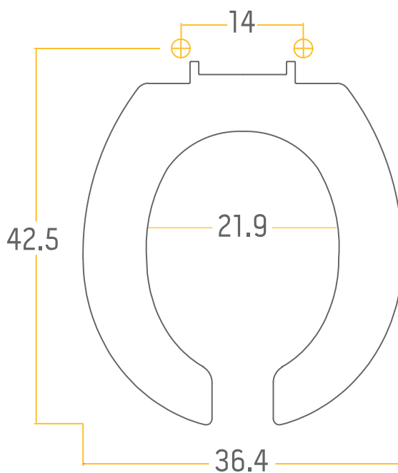
DIMENSIONES
