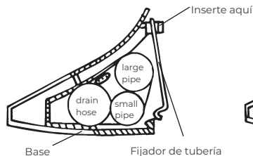
B. Presione para enganchar el fijador de tubería en la base.
