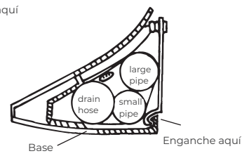
B. Presione para enganchar el fijador de tubería en la base.
